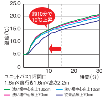
■予備暖房時の浴室内空気温度上昇例
